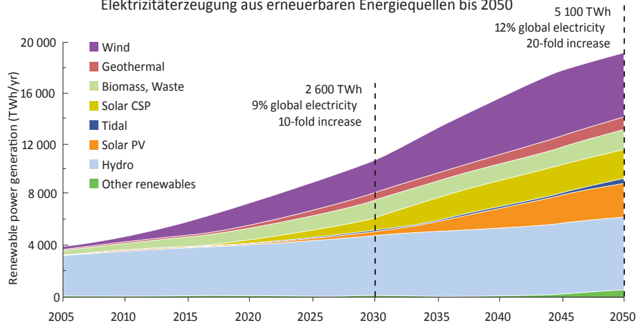
Elektrizitätserzeugung aus erneuerbaren Energiequellen bis 2050
