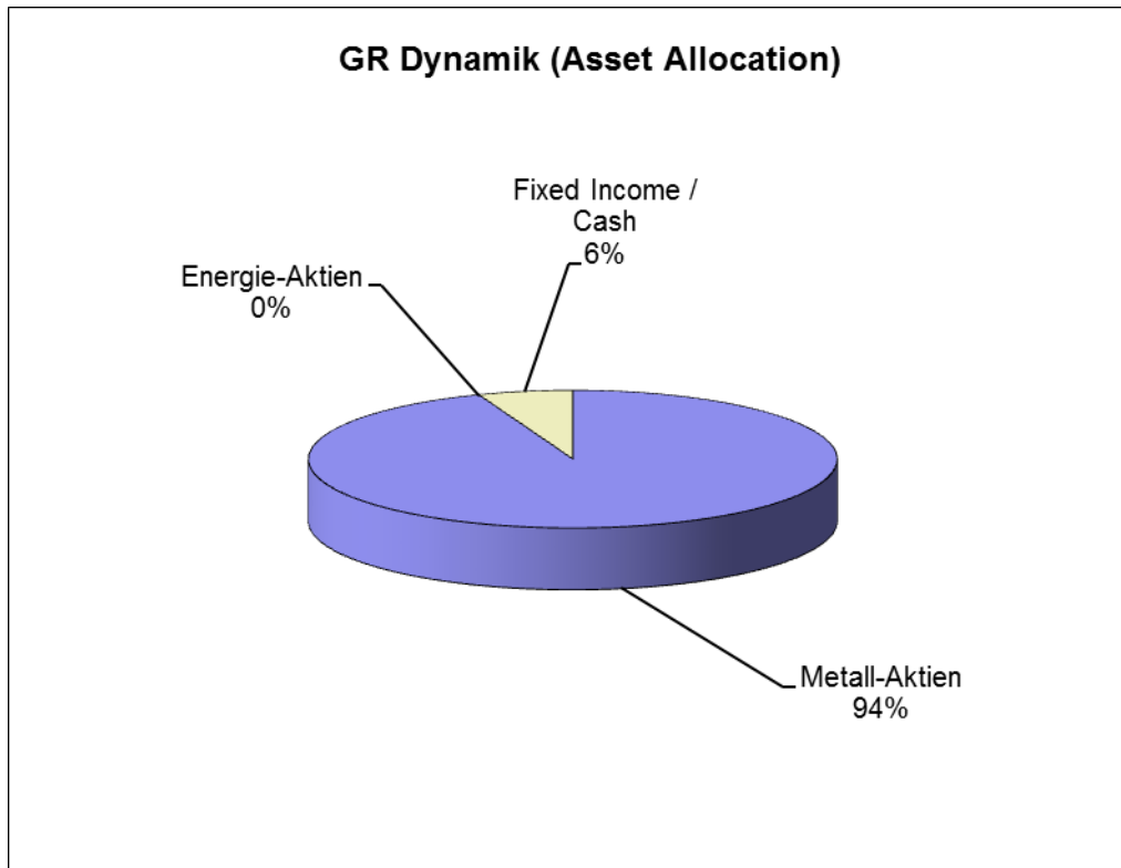
Abb. 3: Asset-Allocation des GR Dynamik (A0H0W9) am 31.10.2015
